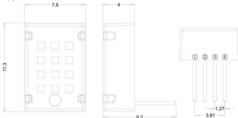
图1 AM2321 外形尺寸
