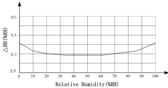
图 2: 25°C 时 AM2321 的相对湿度最大误差
