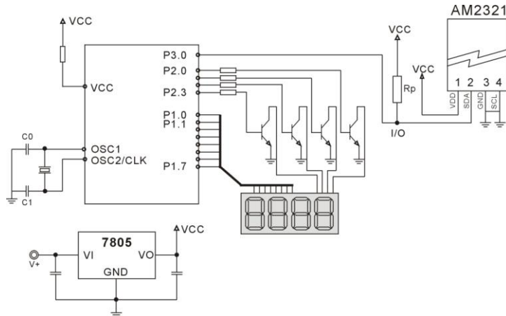
图 19: AM2321 单总线典型电路
